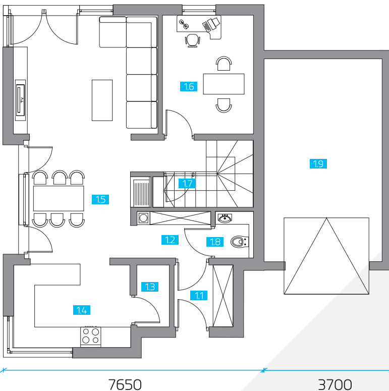
PŮDORYS PŘÍZEMÍ
