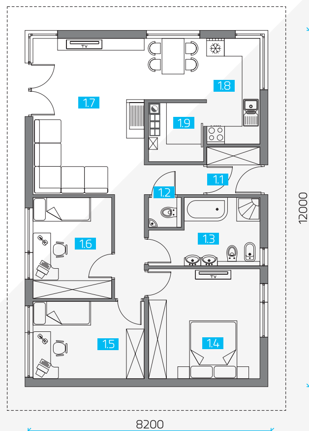
PŮDORYS PŘÍZEMÍ
