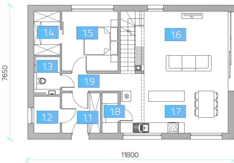
PŘÍZEMÍ
