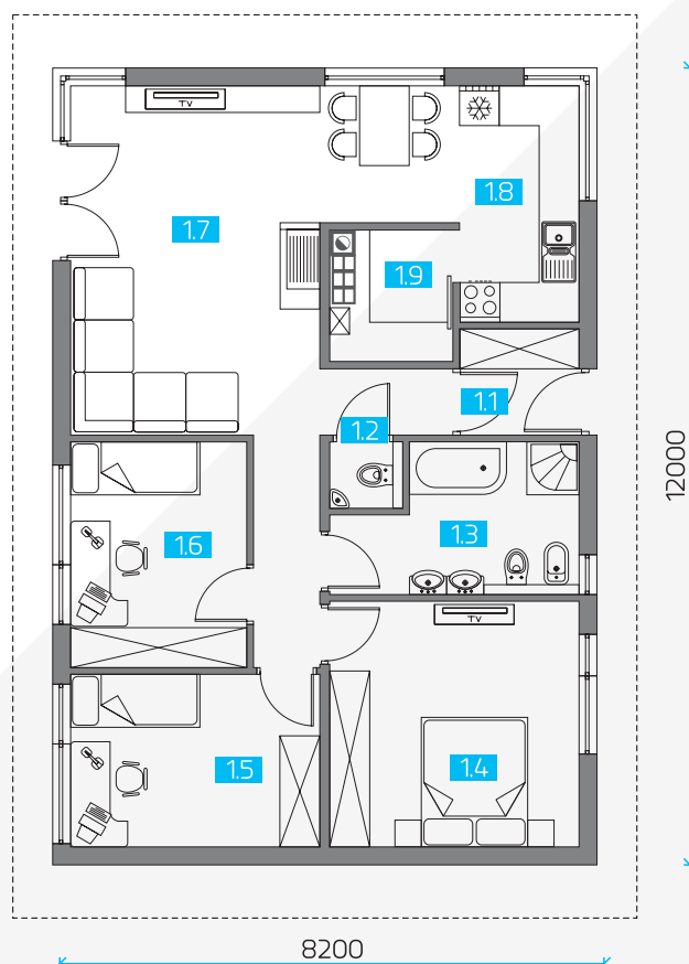
PŮDORYS PŘÍZEMÍ
