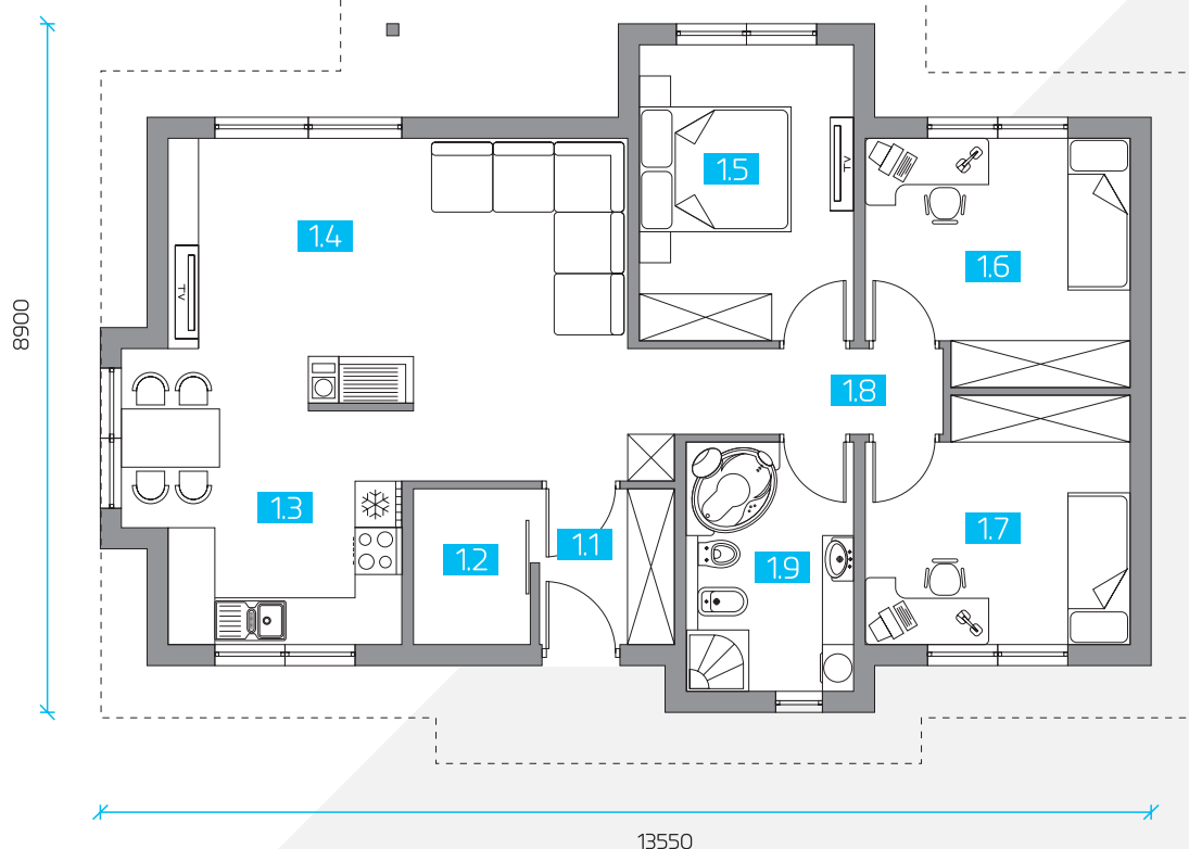
PŮDORYS PŘÍZEMÍ
